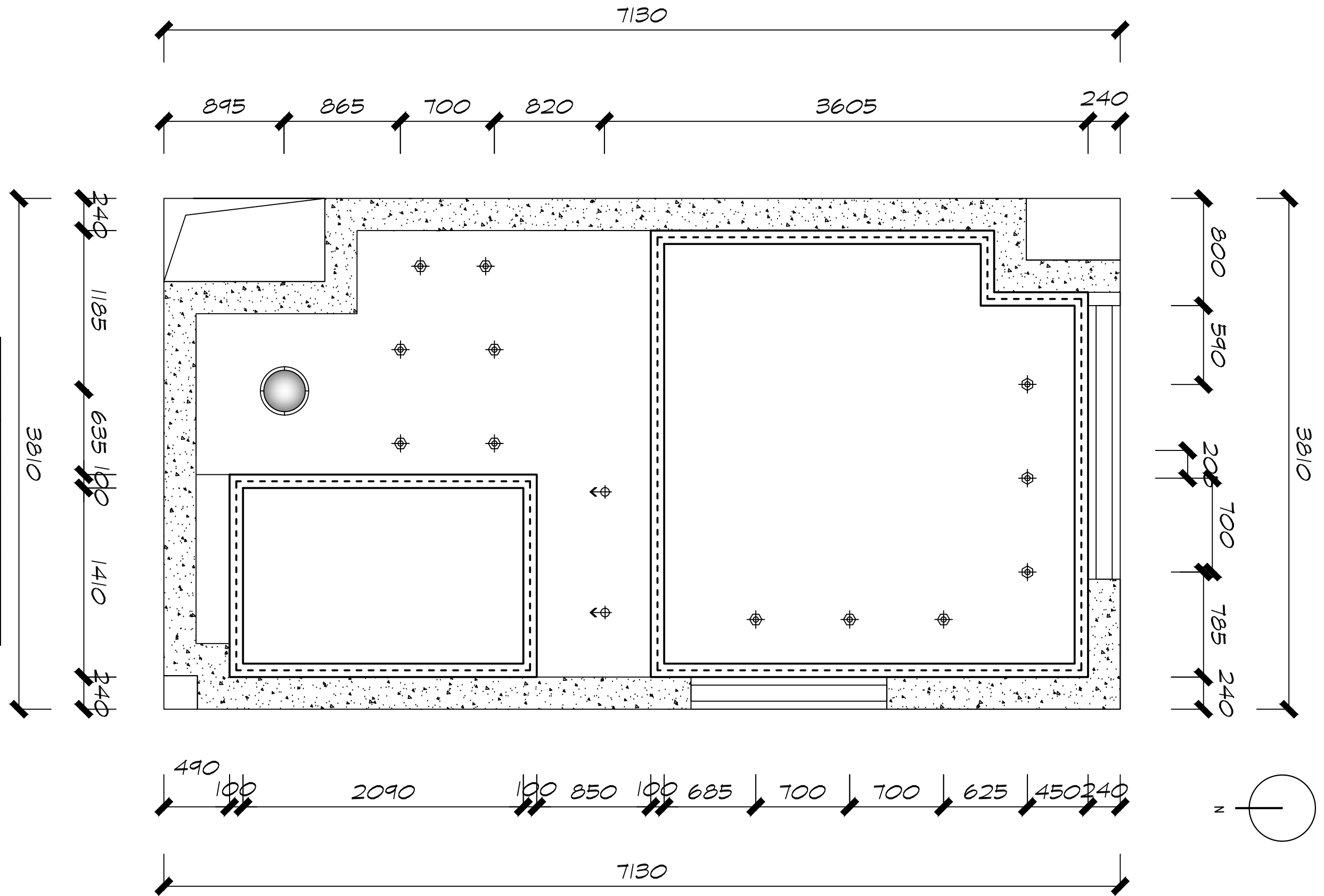
二层天花吊顶图
