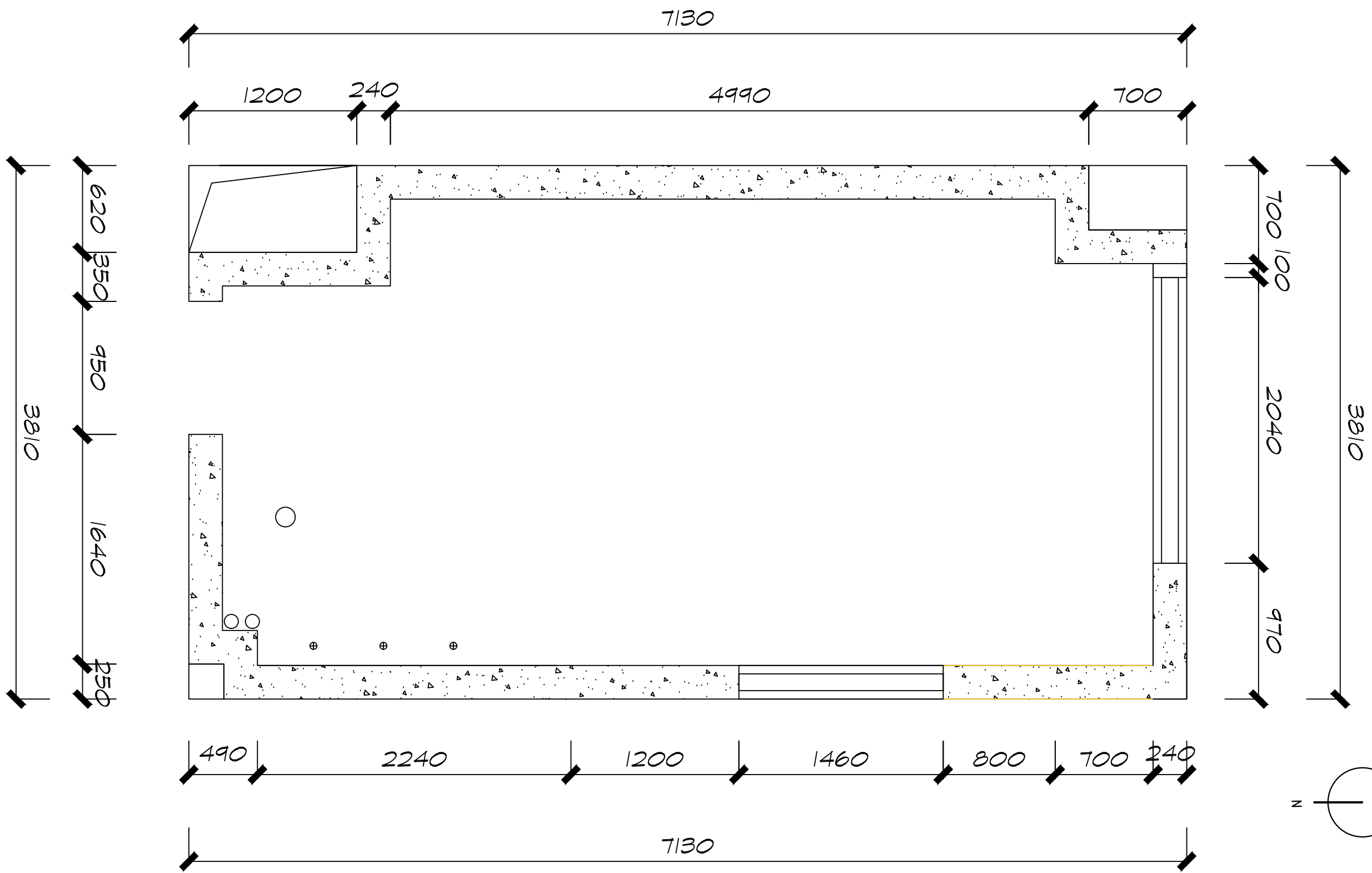
原始平面图 1:30
