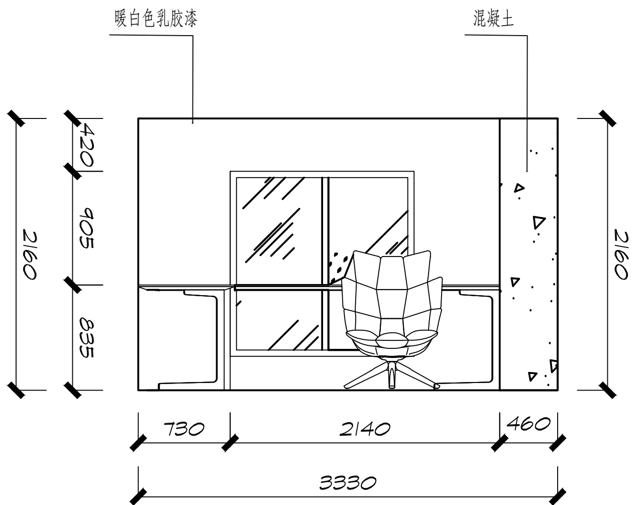
1 2 二层立面图 1:30
