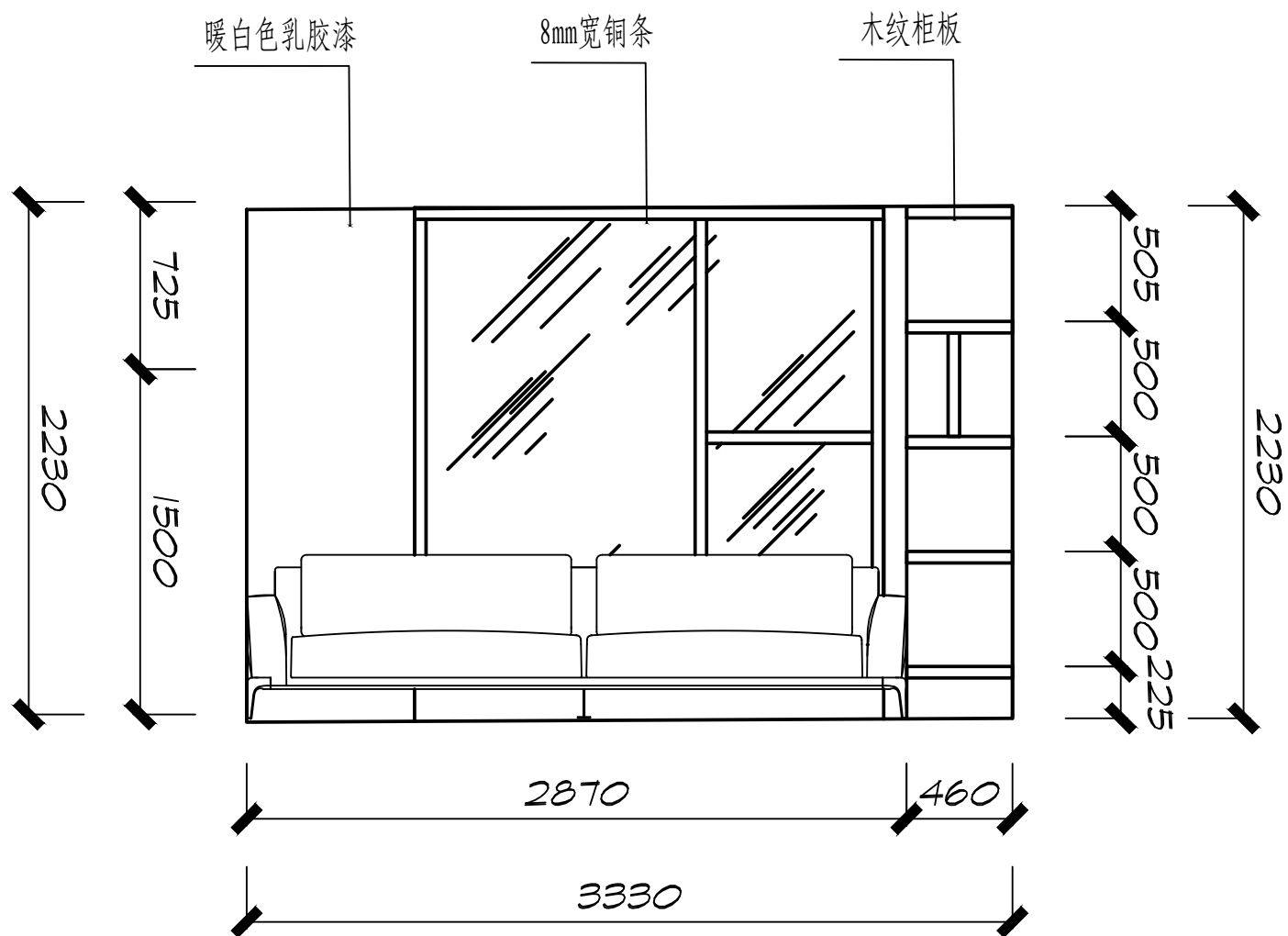
1 1 一层立面图 1:30
