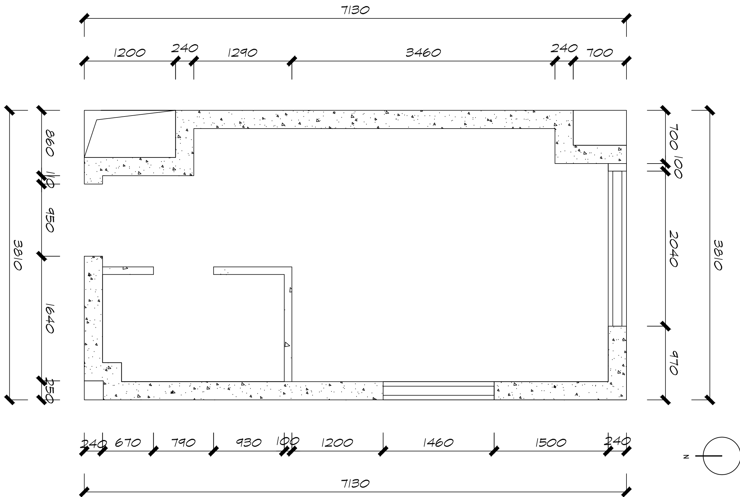
新建墙体图
