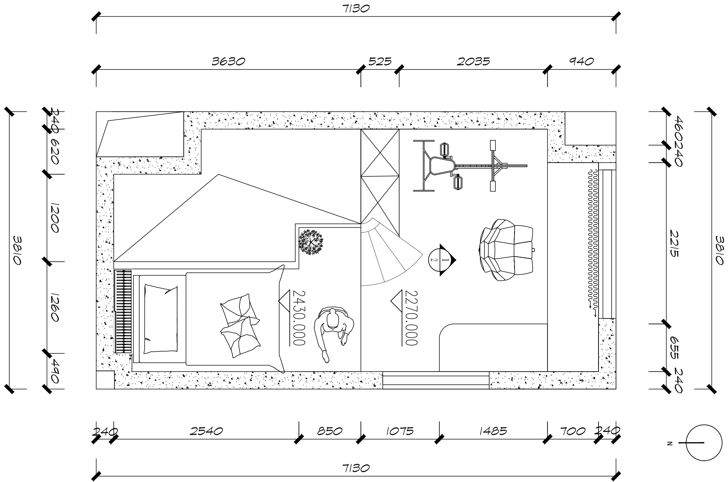
二层平面布置图
